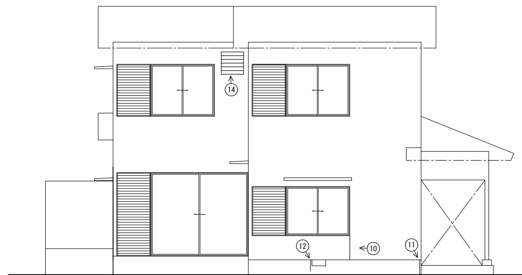
東面 立面図S=1:100
